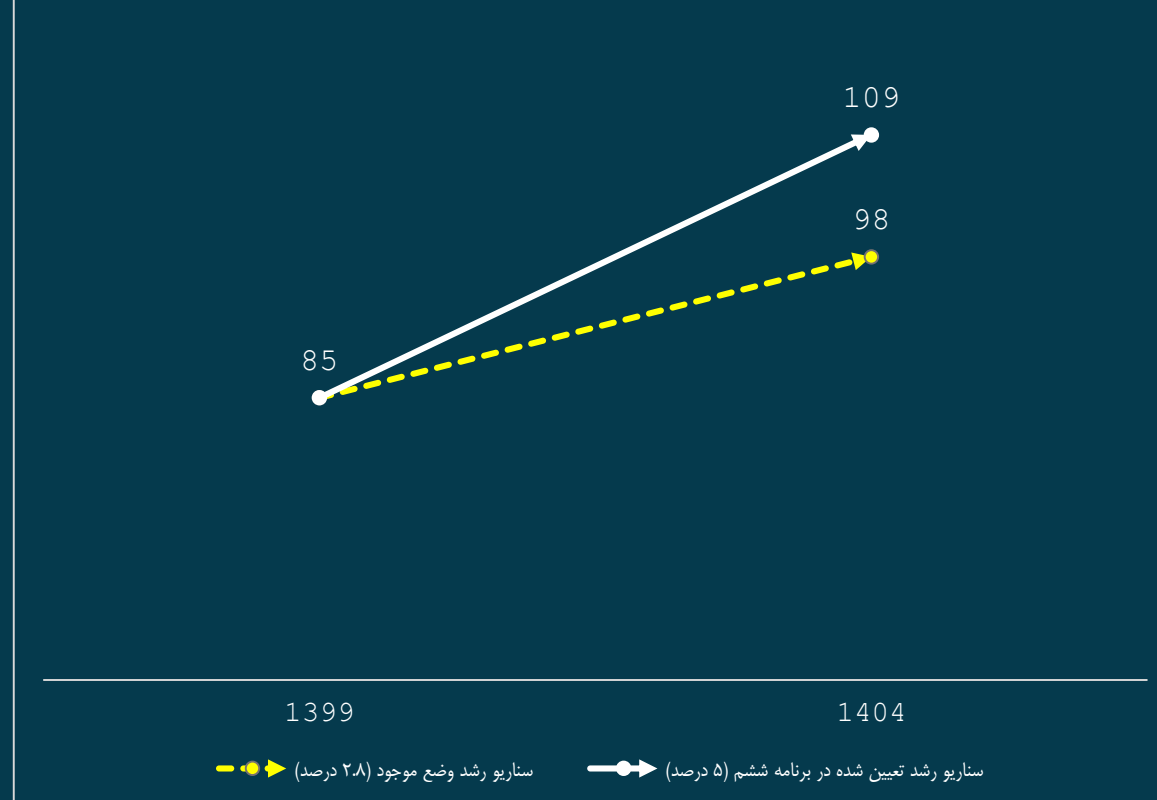
چشم انداز ظرفیت تولید برق کشور در سال ۱۴۰۴ - هزار مگاوات
